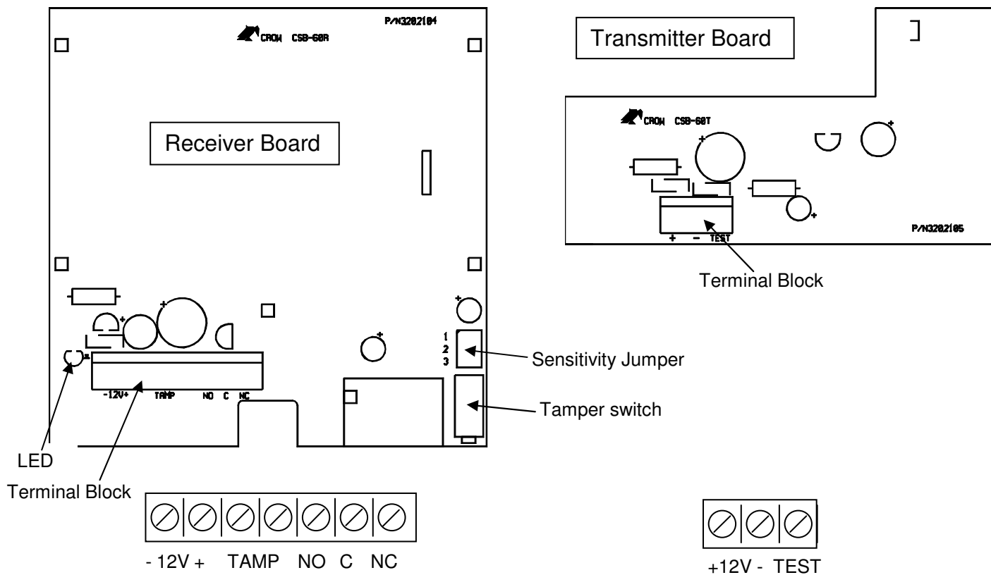
Fig. 5. PCB Layout.
